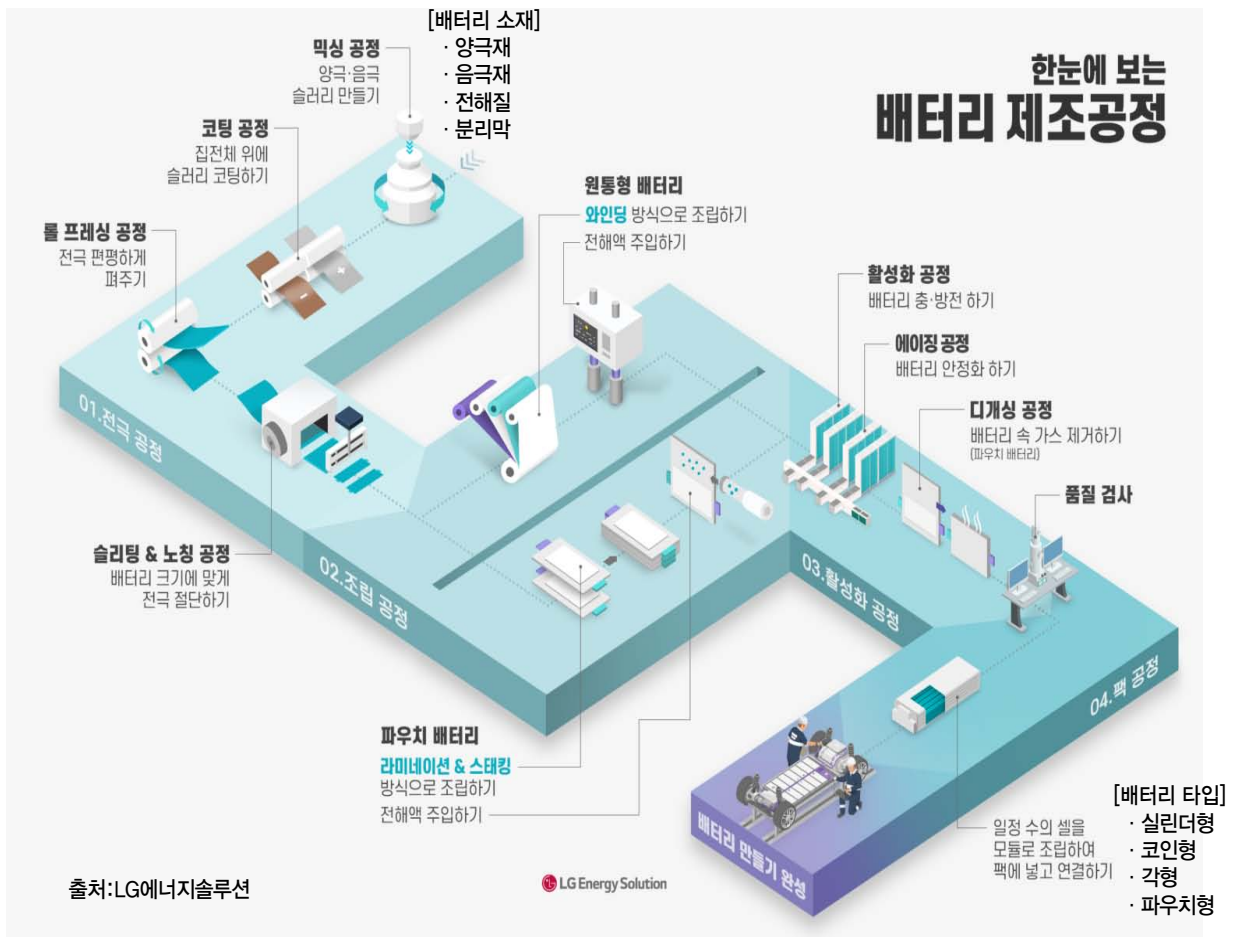
그림 1. 배터리 제조공정 개념도
