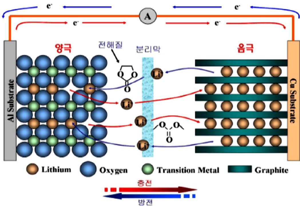
그림 3. 리튬이온 이차전지의 구조 및 작동원리
